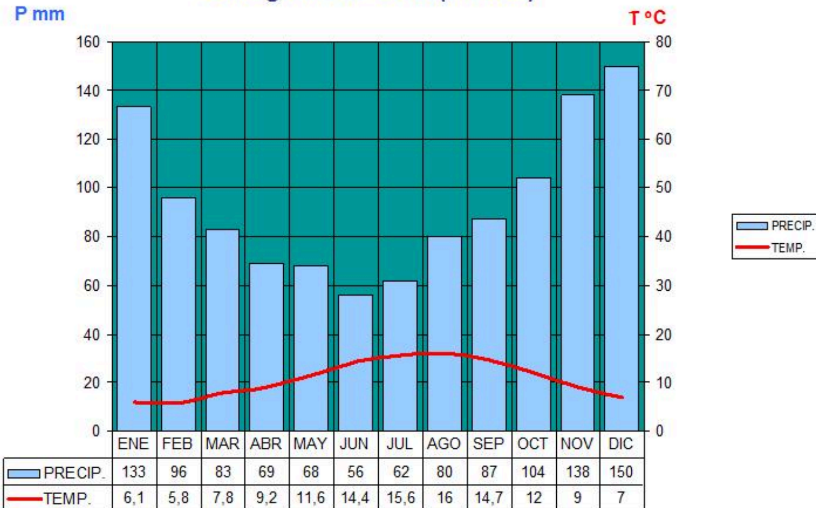
Climograma de Brest (Francia)
