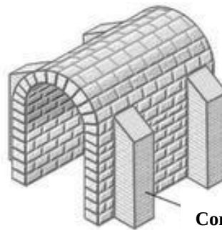
Bóveda de canón
