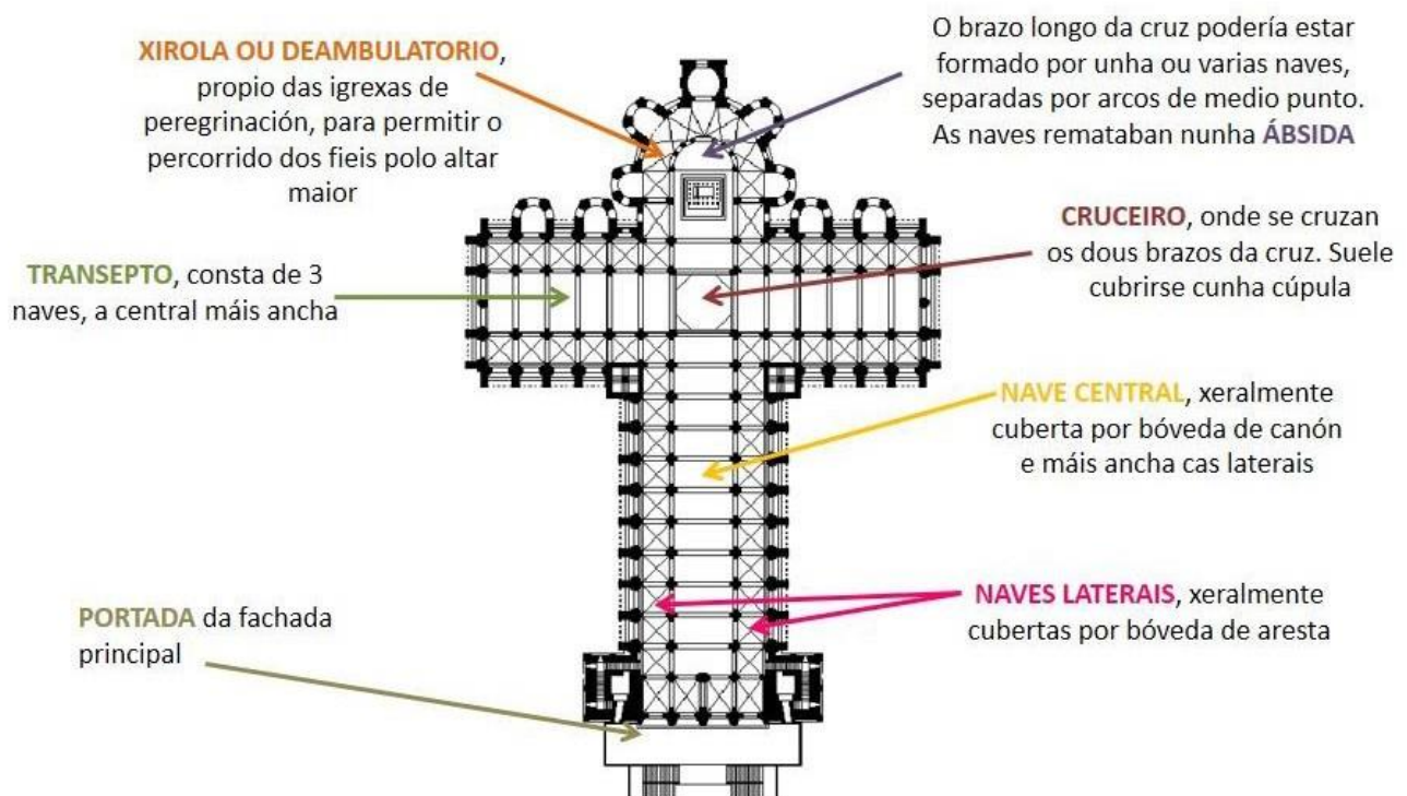
Planta da Catedral de Santiago de Compostela (1075-1211)
