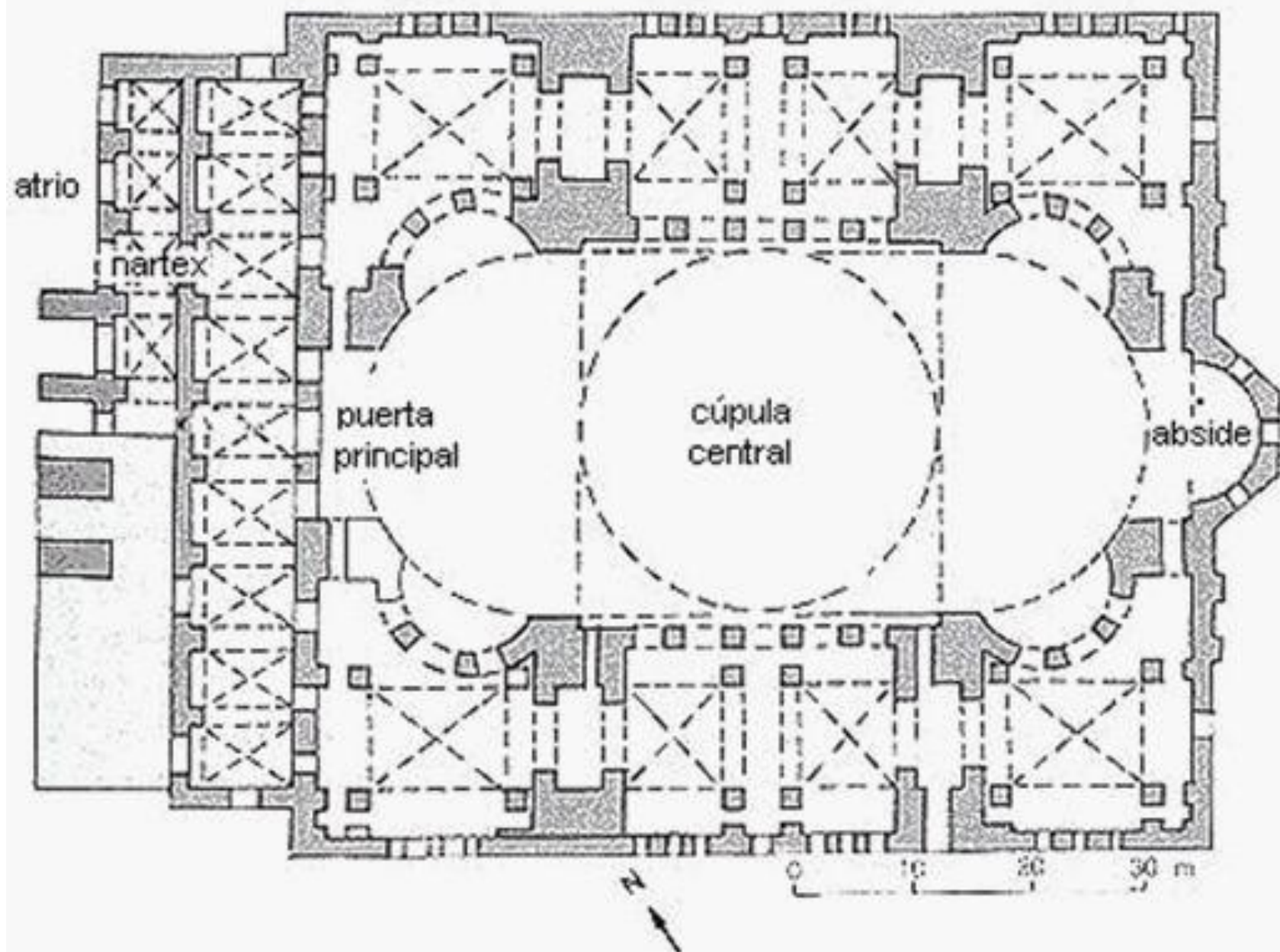
Planta de la Iglesia Santa Sofia
