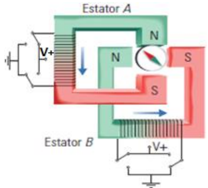
MOTOR PASO A PASO BIPOLAR
