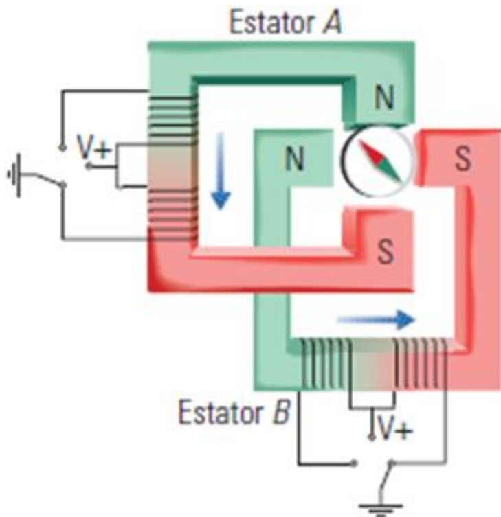
MOTOR PASO A PASO UNIPOLAR
