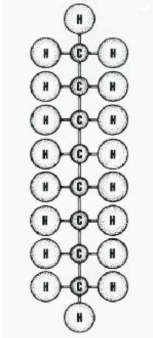
Molécula de hidrocarburo: octano
