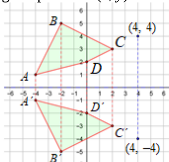
Simetría respecto del eje OX
