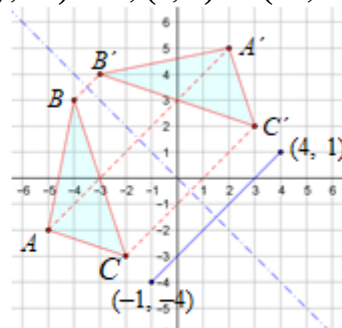
Simetría respecto de la bisectriz del segundo cuadrante
