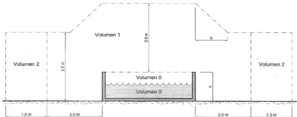
Figura 2. Dimensiones de los volúmenes para depósitos por encima del suelo
