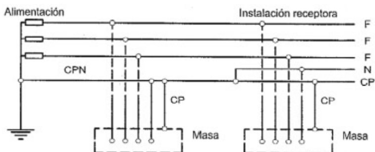
Figura 3. Esquema de distribución tipo TN-C-S
