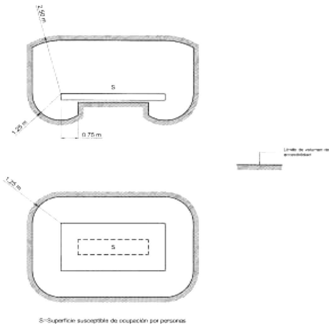
Figura 1. – Volumen de accesibilidad
