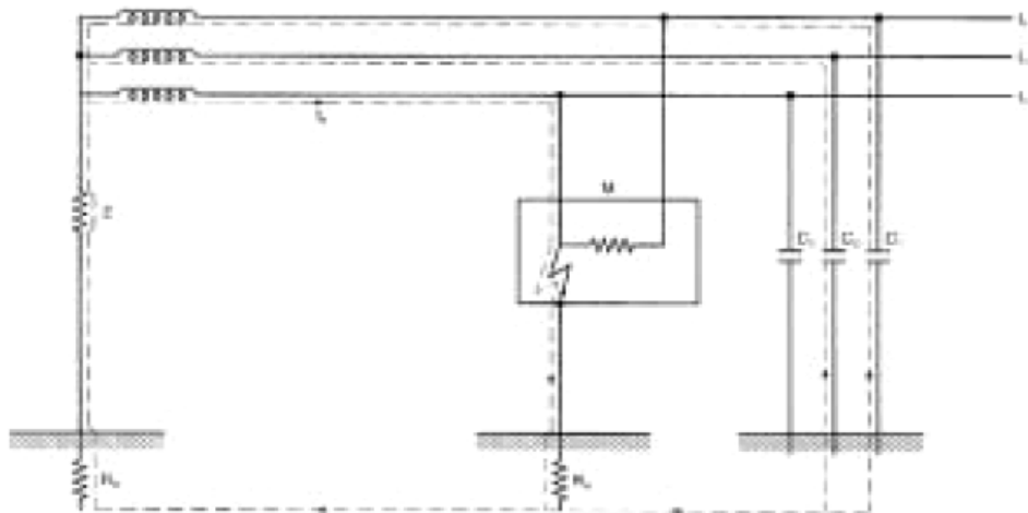
Figura 6. Esquema IT unido a tierra por impedancia Z y con las puestas a tierra de la alimentación y de las masas separadas
