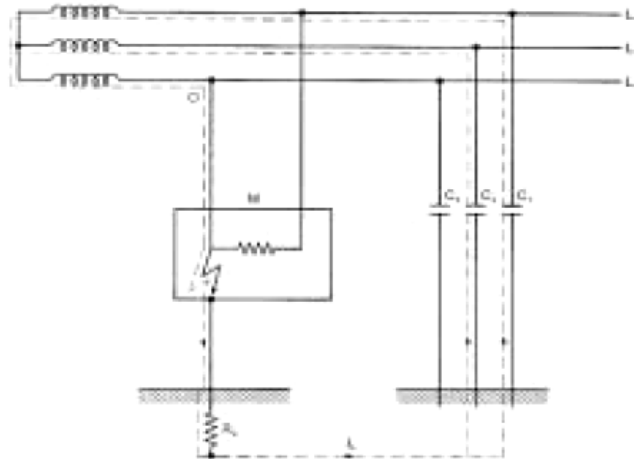
Figura 5. Esquema IT aislado de tierra.
