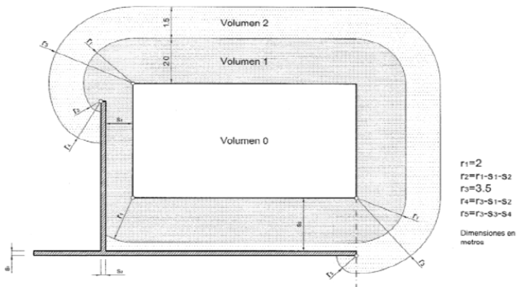
Figura 4. Volúmenes de protección en piscinas con paredes
