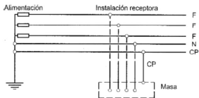
Figura 1. Esquema de distribución tipo TN-S
