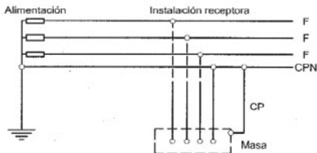
Figura 2. Esquema de distribución tipo TN-C
