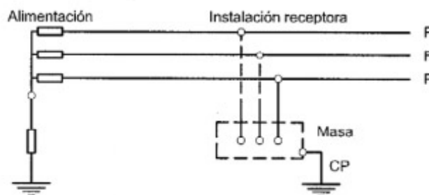
Figura 5. Esquema de distribución tipo IT
