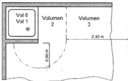
Figura 4 – DUCHA CON PARED FIJA
