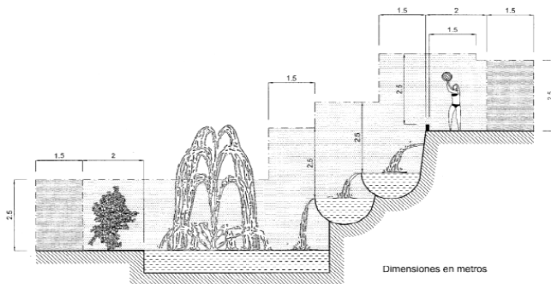
Figura 5. Volúmenes de protección en fuentes
