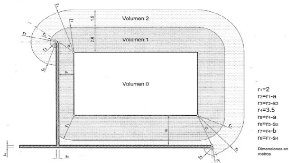
Figura 4. Volúmenes de protección en piscinas con paredes
