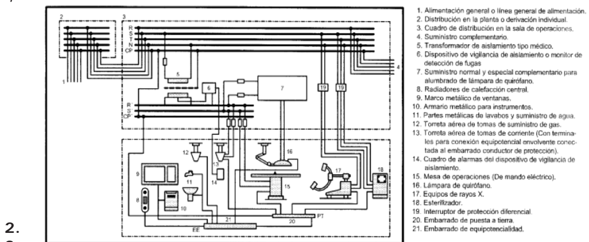
Figura 1. Ejemplo de un esquema general de la instalación eléctrica de un quirófano.
