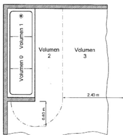
Figura 2 – BAÑERA CON PARED FIJA
