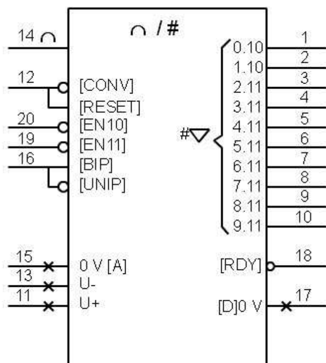
Convertidor analógico-digital (CAD). Ejemplo: AD573
