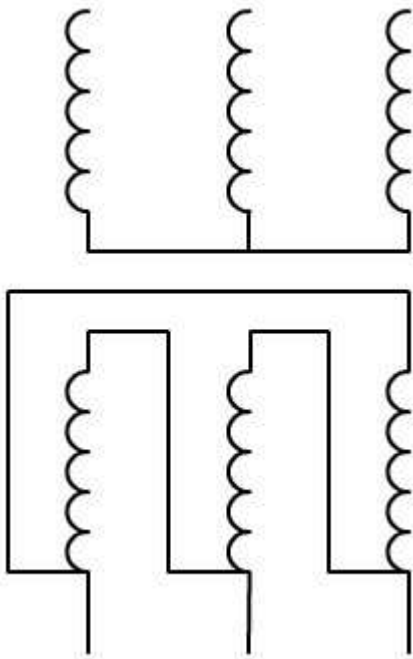
Transformador trifásico, conexión estrella - triángulo. Multifilar
