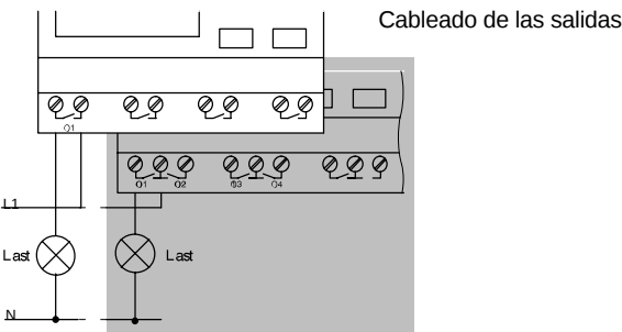
Cableado de las salidas en un LOGO...L...
