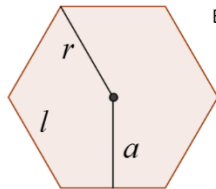
Polígono regular
