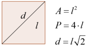
Cuadrado
