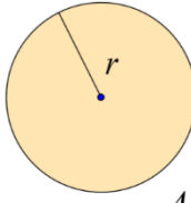
Círculo
