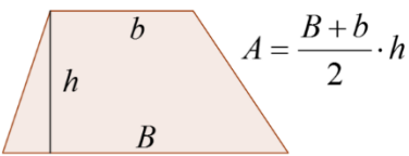
Trapezio
