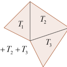
Polígono
