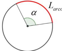
Arco
