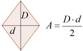
Rombo
