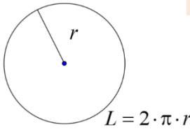
Circunferencia
