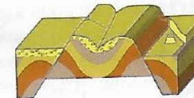
A erosión reactivase e actúa de forma diferencial desgastando primeiro os materiais máis brandos.
