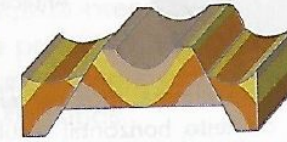
Resultado: relevo de serras longas, paralelas e de altitude similar nos materiais duros, separadas por vales abertos nos estratos brandos.
