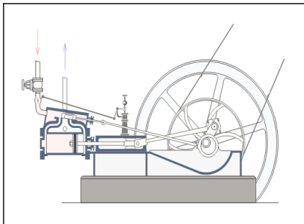
Máquina de vapor
