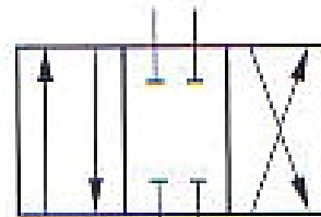
4/3 CC
