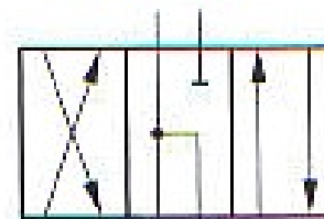
4/3 CD
