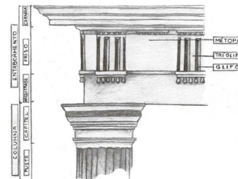
ENTABOAMENTO DÓRICO
