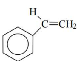
estireno
