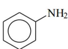
anilina
