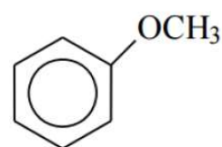
anisol
