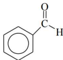
benzaldehído
