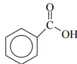
ácido benzoico
