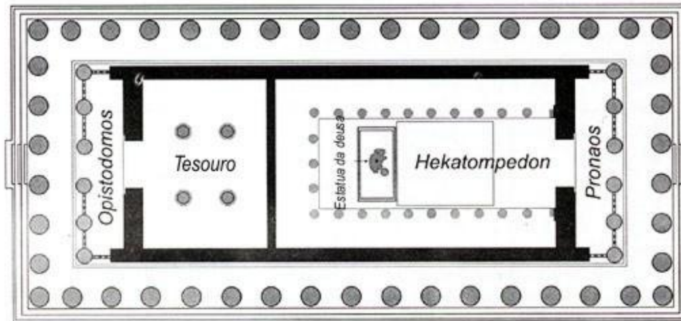
Partenón (planta)
