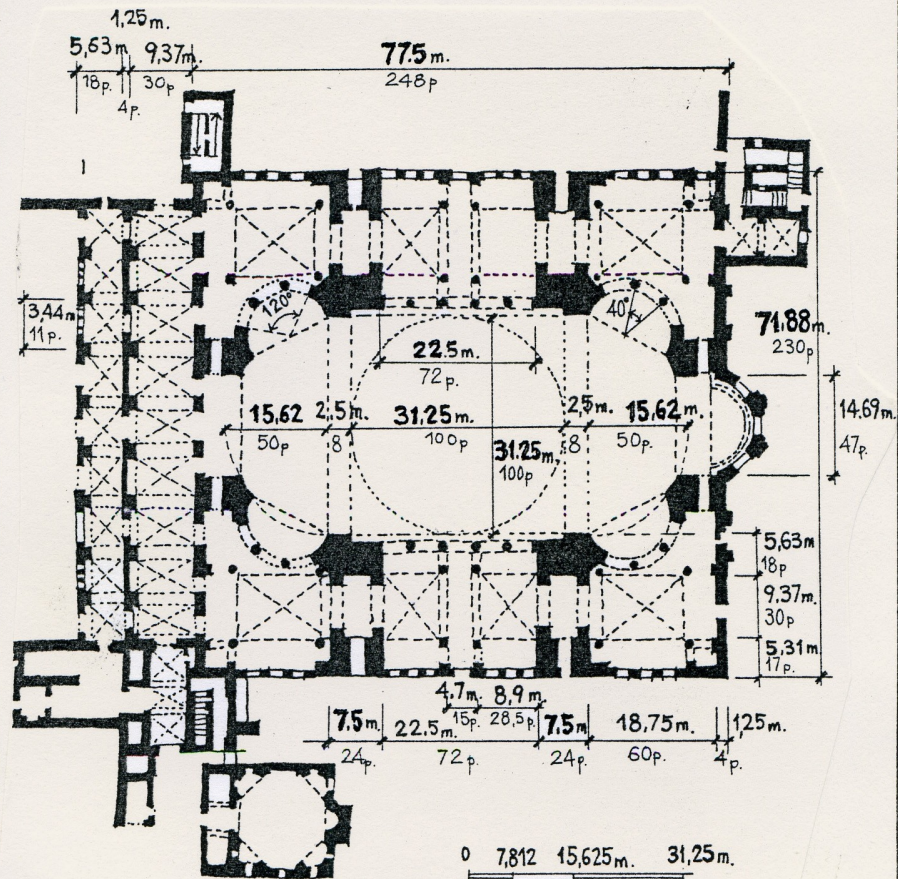
Santa Sofía de Constantinopla. Plano de cotas.
