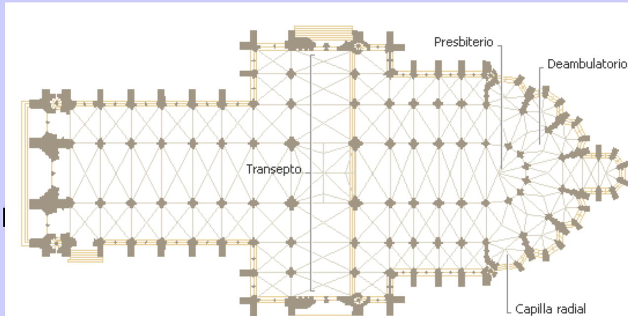
Planta de la catedral de Amiens
