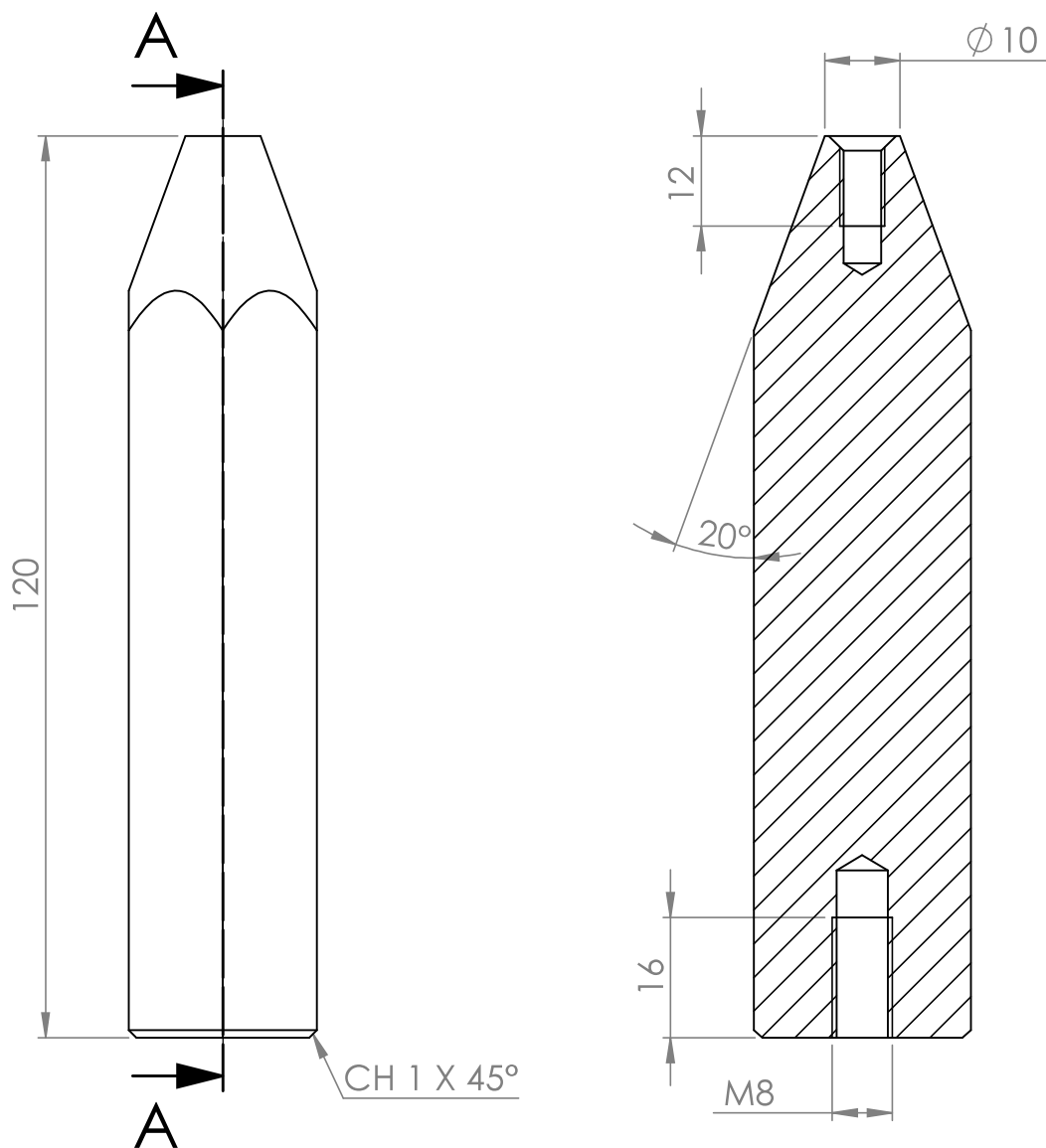
SECCIÓN A-A
