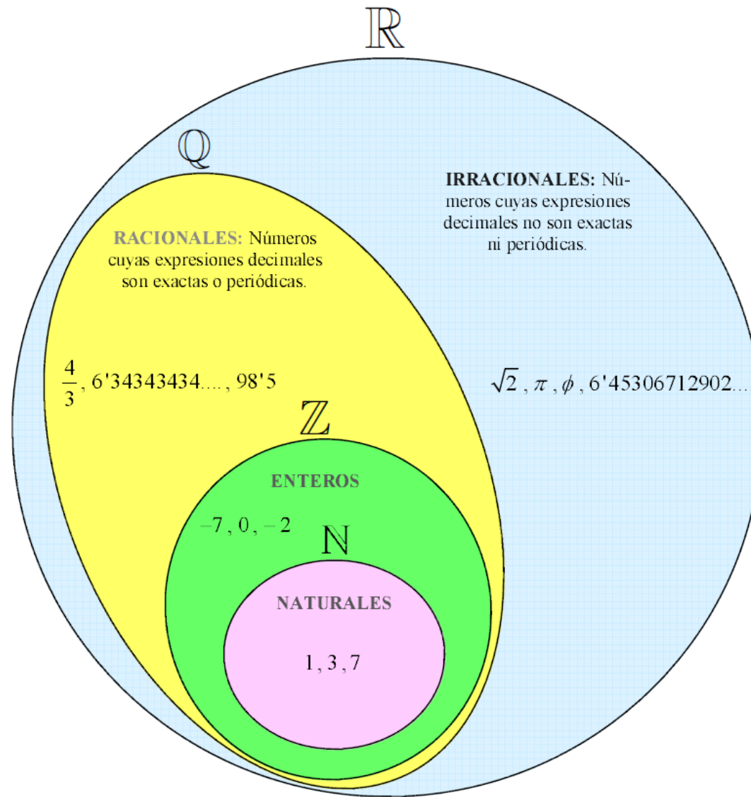
Diagrama de Venn de los números reales
