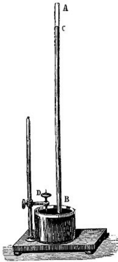
Fig. 276. — baromètre à cuvette et sa pointe.
