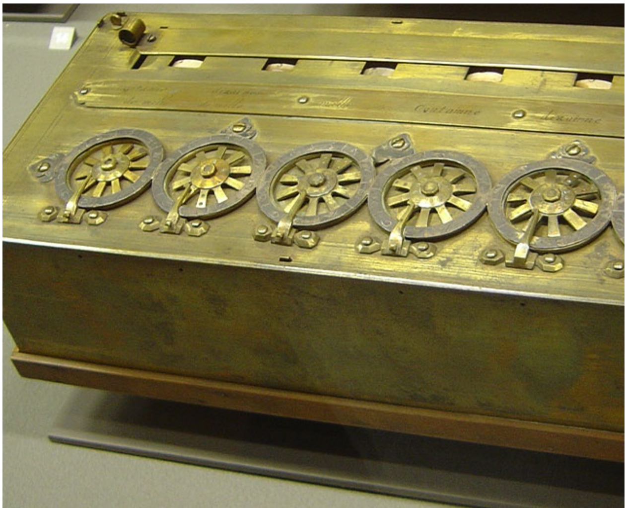
Máquina de cálculo aritmético de Blaise Pascal.
