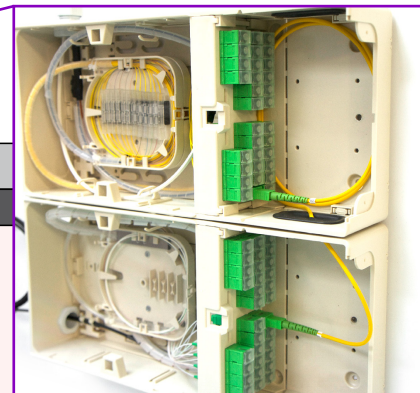
Punto de Interconexión de cables de Fibra Óptica (en RITI)
