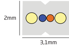
Cable Plano de Acometida Exterior / Interior G657A2. 2 Fibras
