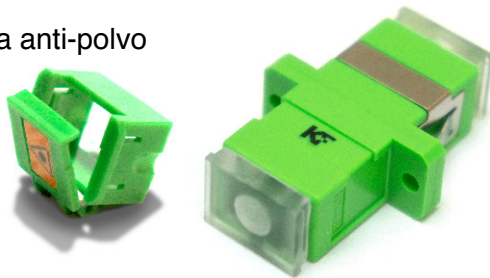
Adaptador SC/APC Tapa transparente
