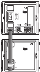
Módulo pulsadores 352100
