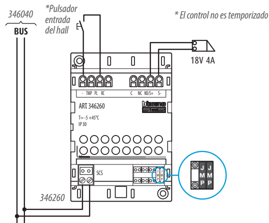
Actuador 346260
