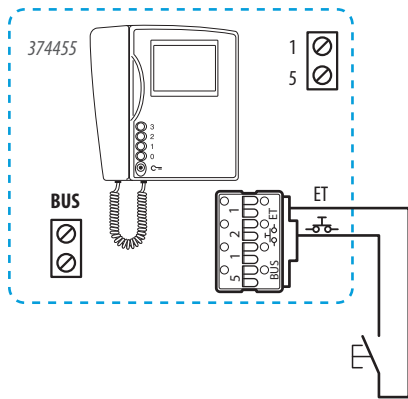
Ejemplo - Conexión del terminal de video SWING
