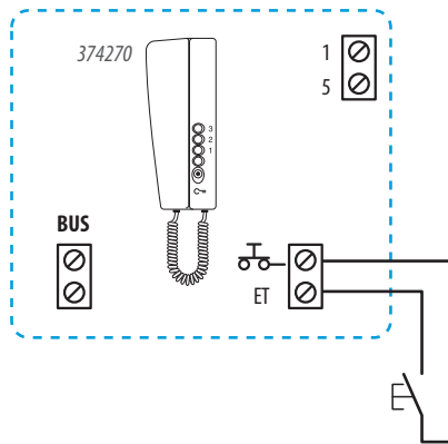
Ejemplo - Conexión del terminal de audio SWING
