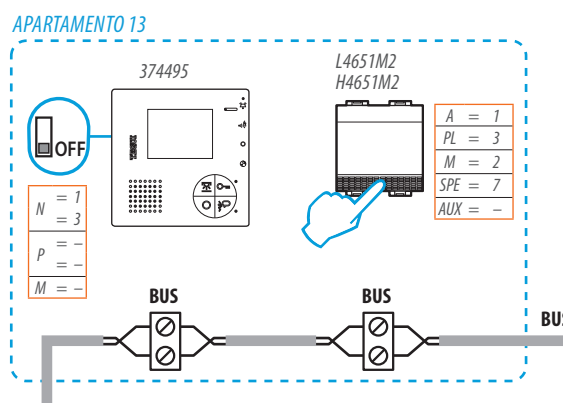
Ejemplo - Llamada a planta en el BUS, conexión después del terminal. Si el control especial está conectado como el último canal o línea del apartamento, se necesita instalar un terminador, elemento 3499, en la ENTRADA-SALIDA en el control.
