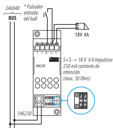
Actuador 346230
