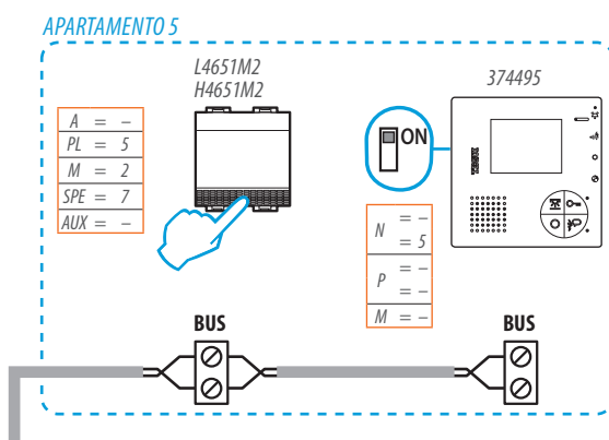
Ejemplo - Llamada a planta en el BUS, conexión antes del terminal.
