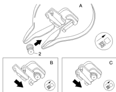
Fig.3 Bloqueo del pivote de sujeción.
