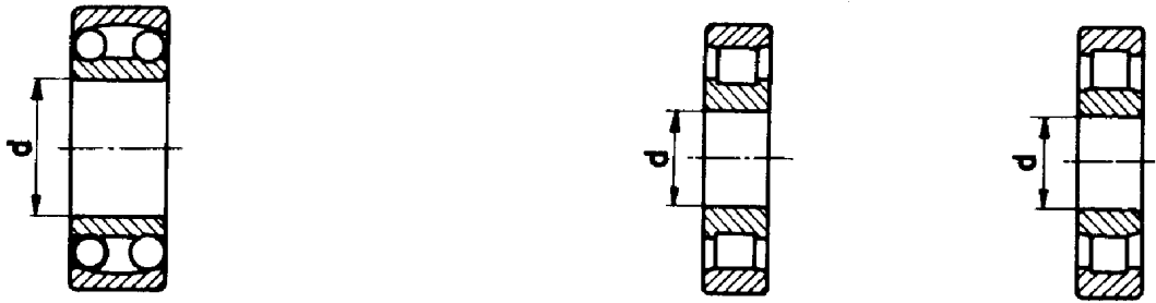
Rodamiento radial oscilante de bolas
