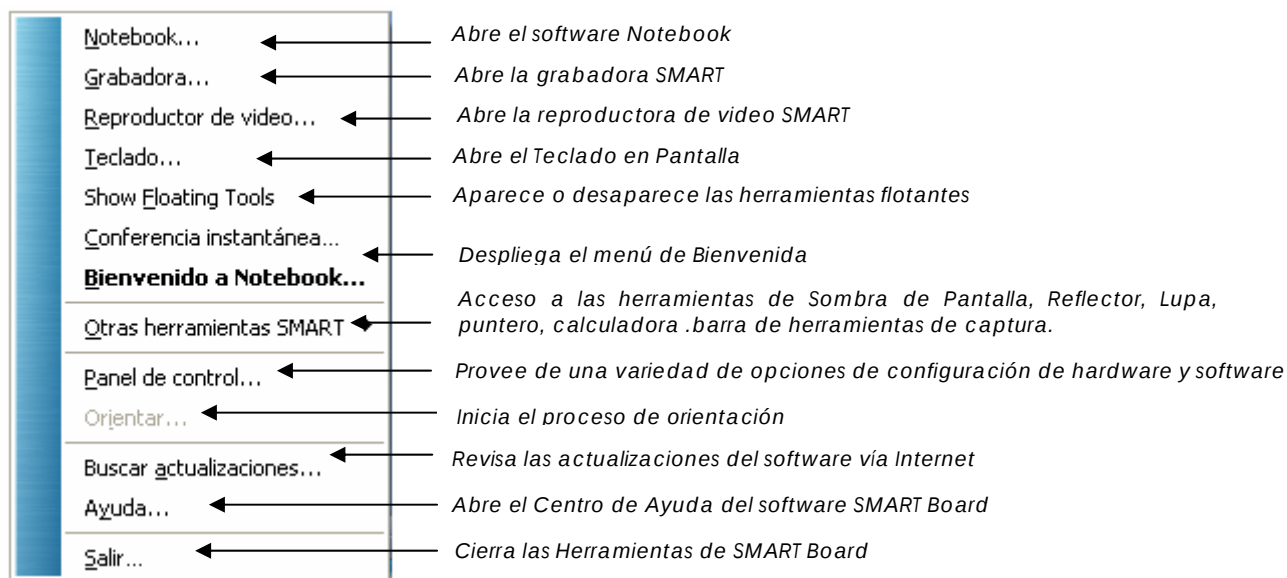
Menú de herramientas de SMART Board
