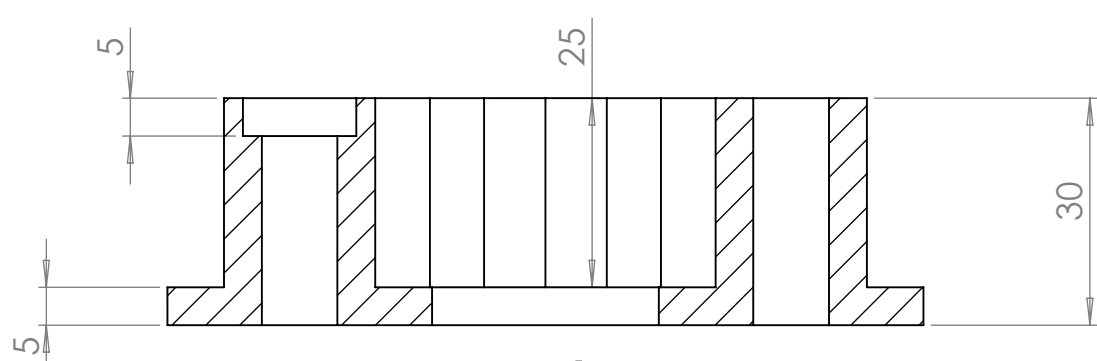
SECCIÓN A-A ESCALA 1 : 1
