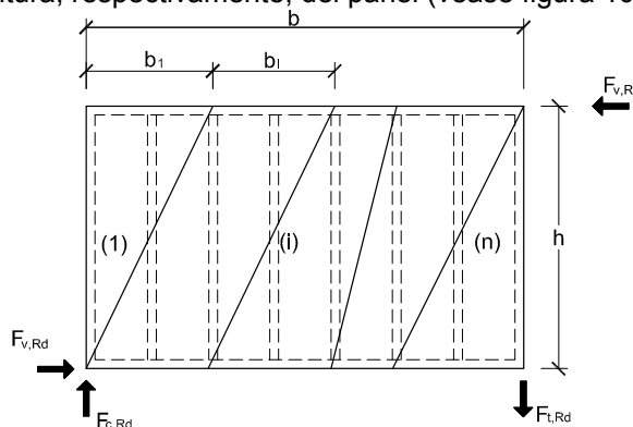
Figura 10.7 Muro diafragma
