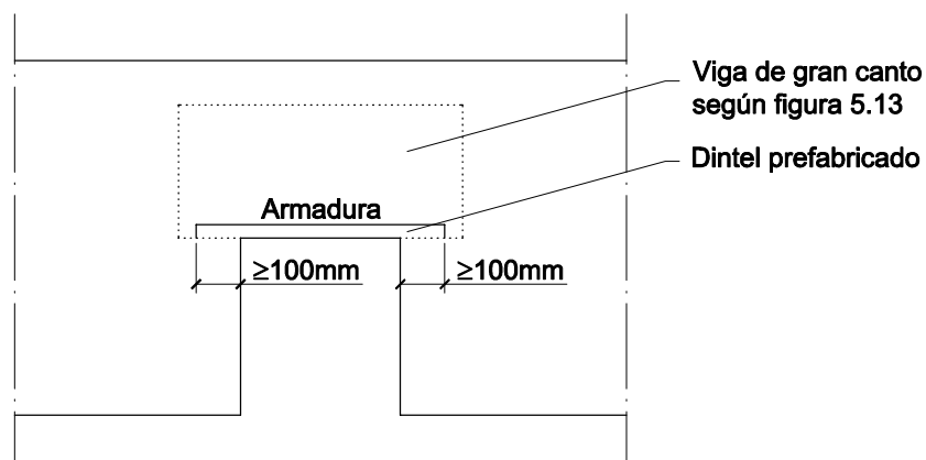
Figura 5.14 Viga de gran canto con dintel compuesto
