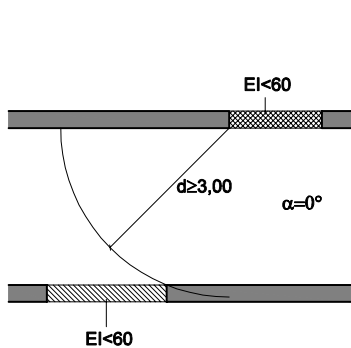
Figura 1.1. Fachadas enfrentadas
