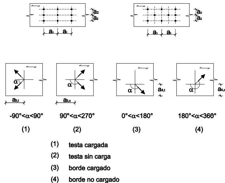
Figura 8.7 Separaciones, distancias y ángulo \alpha .
