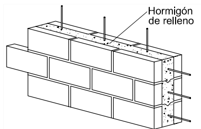
e) Muro relleno de hormigón
