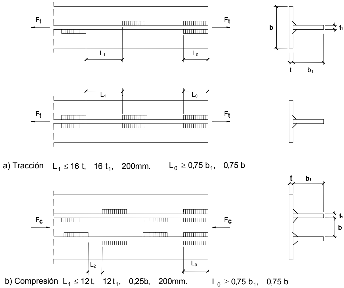
Figura 8.7 Soldadura en ángulo discontinua
