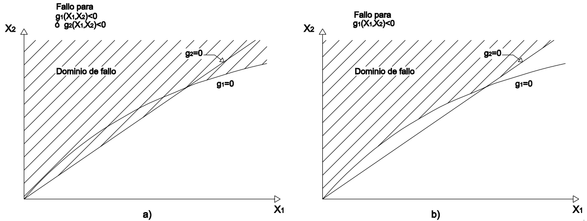
Figura C.2 Dominios de fallo para un ejemplo con dos funciones g_1(X_1, X_2) y g_2(X_1, X_2) con dos variables básicas X_1 y X_2 . a) Fallo del sistema producido por el de una sección; b) Fallo de un sistema redundante
