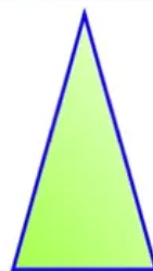
ISÓSCELES
