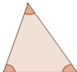
ACUTÁNGULO
