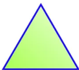
EQUILÁTERO
