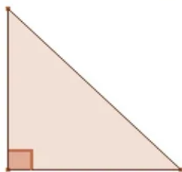
RECTÁNGULO
