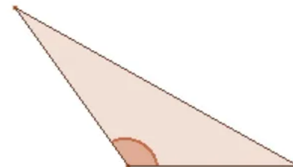
OBTUSÁNGULO
